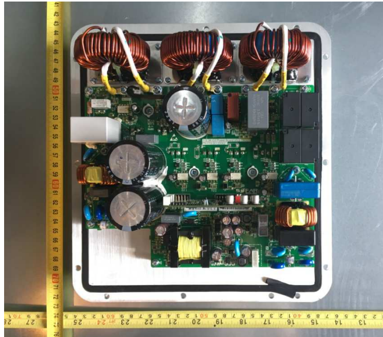
Figura 3. Visão interna-1 Figure 3. Internal view-1
