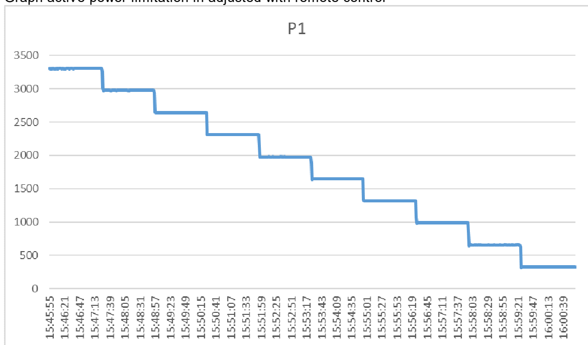
Gráfico limitação da potência activa em coincidência com comando remoto Graph active power limitation in adjusted with remote control
